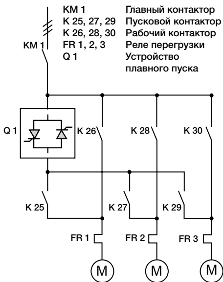
Последовательный пуск двигателей с помощью устройства плавного пуска
