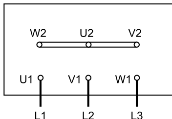
Y - Подключение 400 В (690 В)
