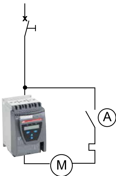
Вариант А Главный контактор находится внутри треугольника
