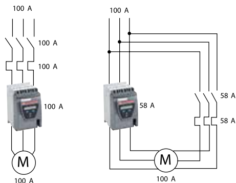
Устройство плавного пуска при подключении в линию Устройство плавного пуска внутри треугольника
