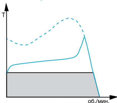
График зависимости крутящего момента от скорости при использовании устройства плавного пуска
