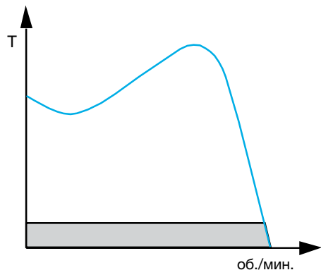
График зависимости крутящего момента от скорости при прямом пуске
