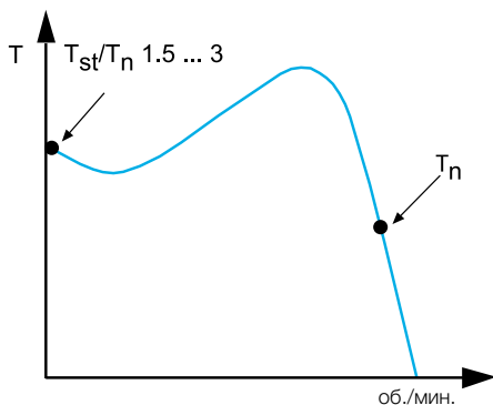
Кривая крутящего момента для двигателя с короткозамкнутым ротором
