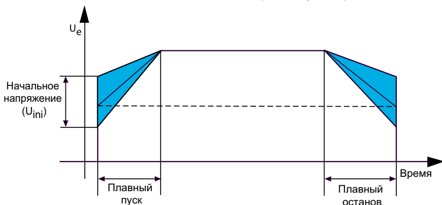
Схема, на которой указано время плавного пуска, останова и начальное напряжение
