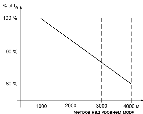
Снижение тока двигателя на больших высотах
