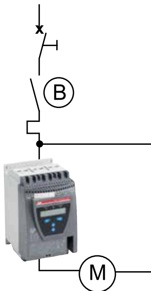
Вариант Б Главный контактор находится за пределами треугольника
