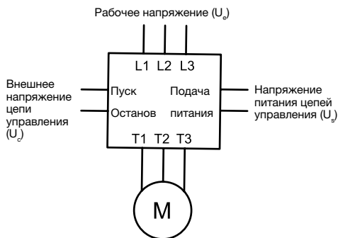
Устройства плавного пуска с внешним напряжением цепи управления
