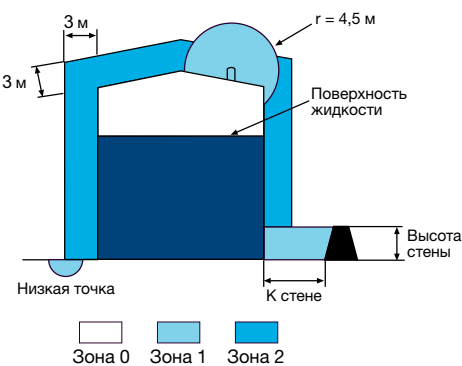
Пример классификации и границы опасных зон в баке
