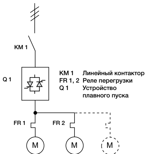
Параллельный пуск двигателей с помощью устройства плавного пуска
