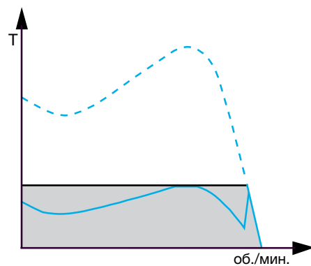
График зависимости крутящего момента от скорости при использовании пускателя со схемой соединения звезда/треугольник
