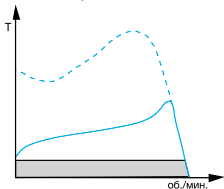
График зависимости крутящего момента от скорости при использовании устройства плавного пуска
