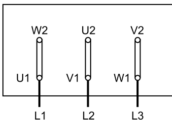
Δ - Подключение 230 В (400 В)
