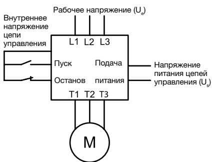
Устройства плавного пуска с внутренним напряжением цепи управления
